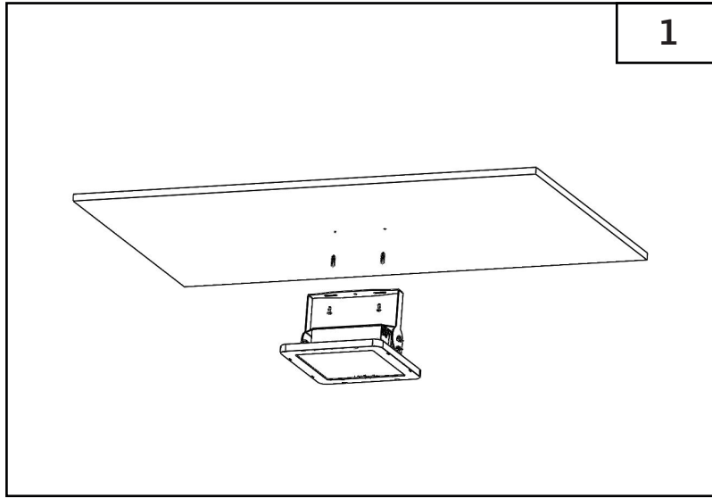
1.1 Armatür askı kolu delikleri tavana hizalanır. 1.1 Luminaire suspension arm holes are aligned with the ceiling.
