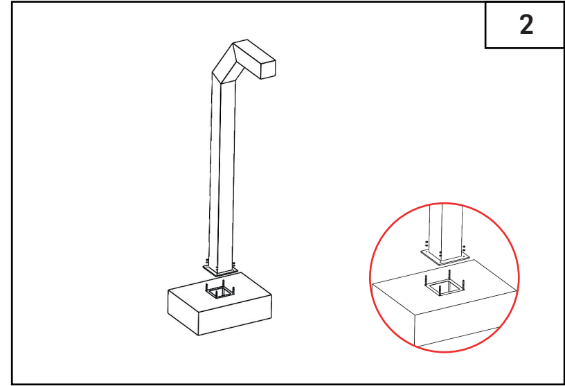
2.1 Armatür ankarağa takılır. 2.1 The armature is attached to the anchor.
