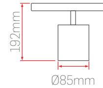
Ağırlık/Weight:1 Kg
